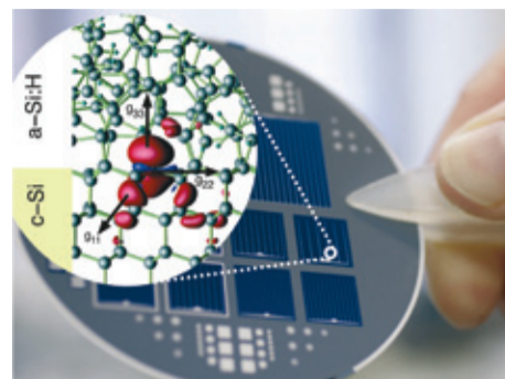
Erkenntnisreiche Fehlersuche: Das Forscherteam vom HZB und der Universität Paderborn konnte erstmals Defekte auf atomarer Ebene von Silizium-Heterokontaktsolarzellen beschreiben. Foto: HZB / Uni Paderborn
